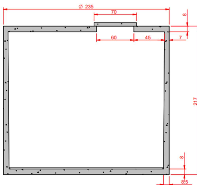
Doorsnede
