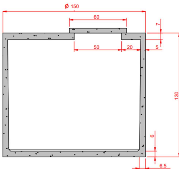
Doorsnede
