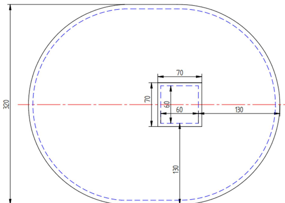
Bovenaanzicht
